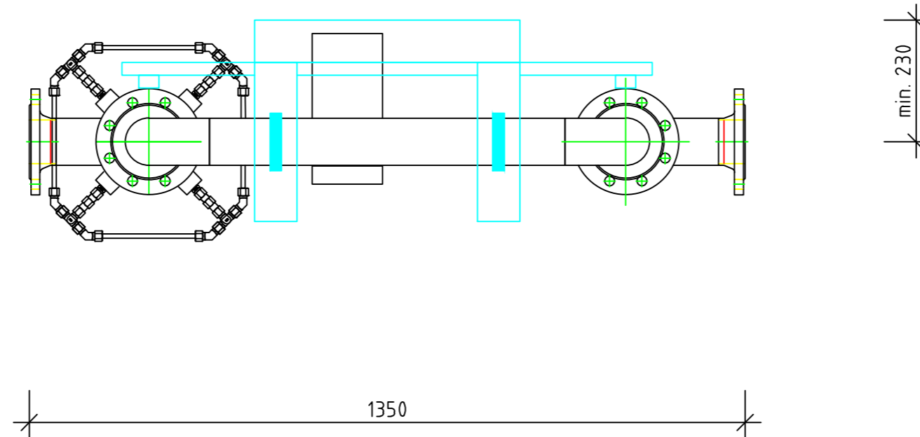
Draufsicht
