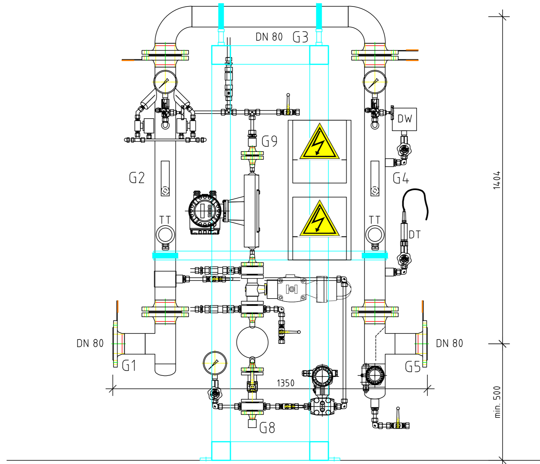
Ansicht - Prolimix
